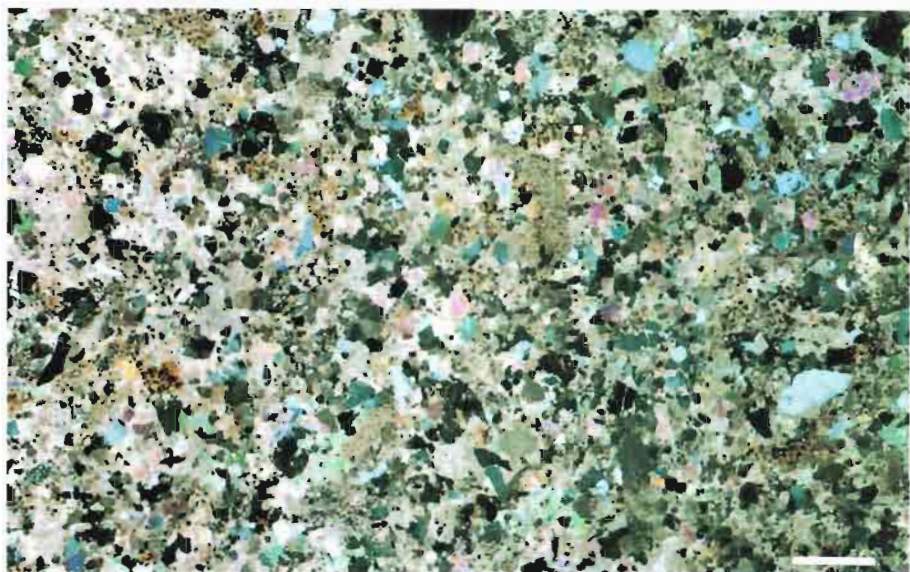
Foto 8. Dolomía arenosa (15-25%) de grano medio a grueso. Los granos de cuarzo están poco redondeados y aparecen parcialmente corroídos por la dolomita. Niveles basales del Mb. Calizas de la Bicuerca. Con nicoles cruzados. Escala 1 mm.
