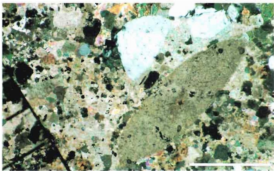
Foto 9. Dolomía arenosa (15-20%) de grano medio a grueso. El bioclasto de gran tamaño, que se encuentra en el centro de la foto, es una sección de una espina de un equinido. Tramos basales del Mb. Calizas de la Bicuerca. Con nicoles cruzados. Escala 1 mm.
