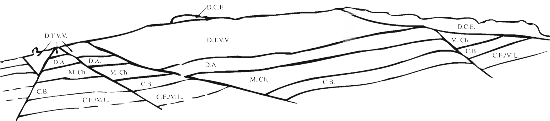
Vista del frente occidental del Cerro del Bosque. Relaciones verticales y laterales de las unidades descritas.
