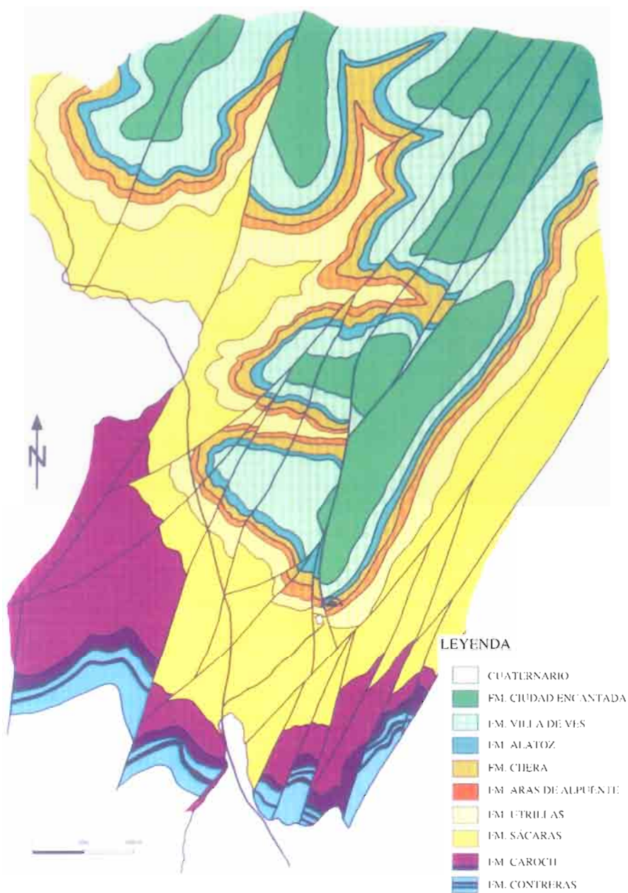
Figura 6. Cartografía geológica de detalle del Cerro del Bosque.
