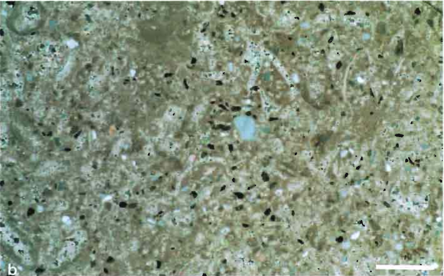
Foto 5. Packstone arenoso. Fragmentos de conchas recristalizadas de pelecípodos y pellets. Granos de cuarzo de tamaño arena fina. Parte media de la Fm. Sácaras.
