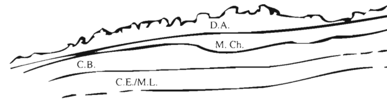
C.E./M.L.: Mbs. Estenas y Losilla. C.B.: Mb. Bicuerca. M.Ch.: Fm. Chera D.A.: Fm. Alatoz. D.T.V.V.: Fm. Villa de Ves. D.C.E.: Fm. Ciudad Encantada
