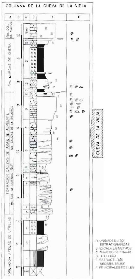
Figura 7. Columna estratigráfica detallada de la Cueva de la Vieja.
