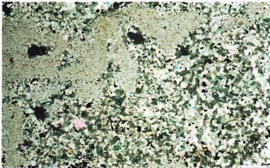
Foto 12. Dolosparita que presenta dos modas bien diferenciadas en el tamaño cristalino. Las zonas (parches) con menor tamaño, corresponden a tubos de bioturbación. Tramos basales de la Fm. Dolomías de Alatoz. Con nicóles cruzados. Escala 1 mm.
