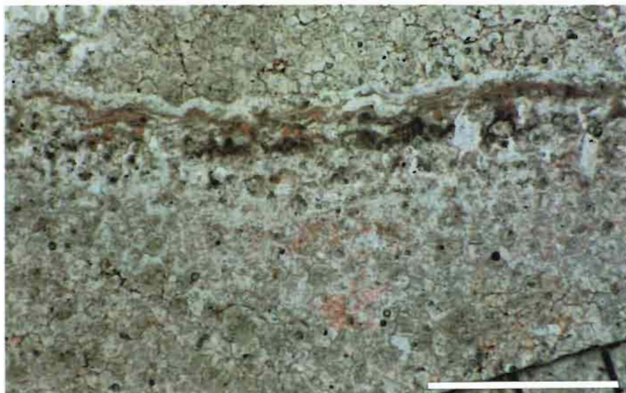
Foto 19. Doloesparita mesocrystalina , ligeramente limosa. En la mitad superior de la fotografía se observa una fisura parcialmente rellenada por un cemento de tipo espeleotema. Los niveles de carácter micrítico podrían reflejar la actividad de microorganismos. Escala 1 mm.
