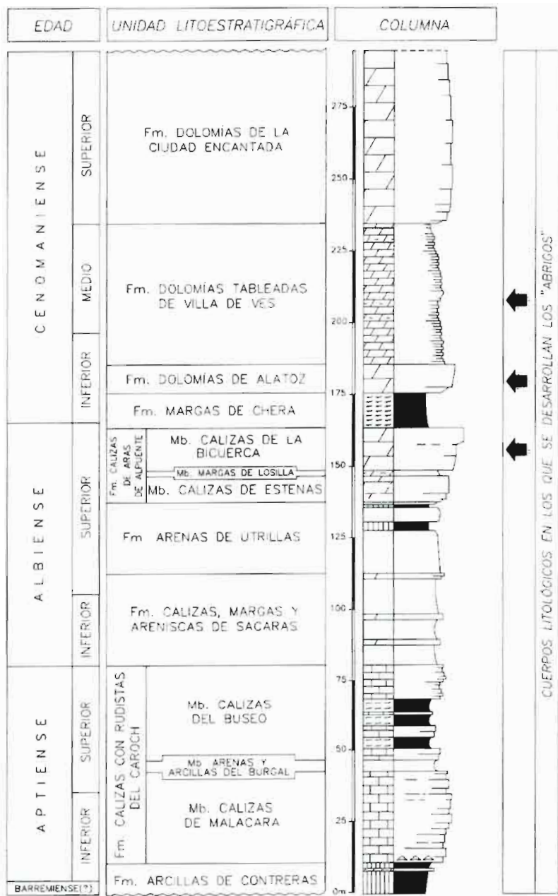
Figura 5. Columna estratigráfica general del Cretácico de la Muela de Alpera.
