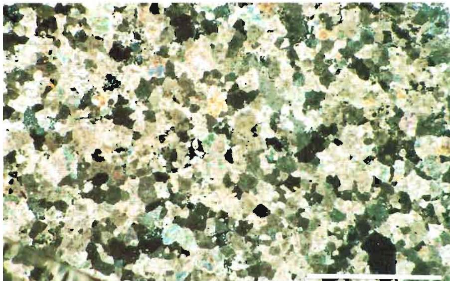
Foto 6. Dolosparita mesocristalina, formada por cristales subeuhedrales homométricos, de contactos rectos. Tramos altos del Mb. Calizas de la Bicuera. Con nicóles cruzados. Escala 1 mm.
