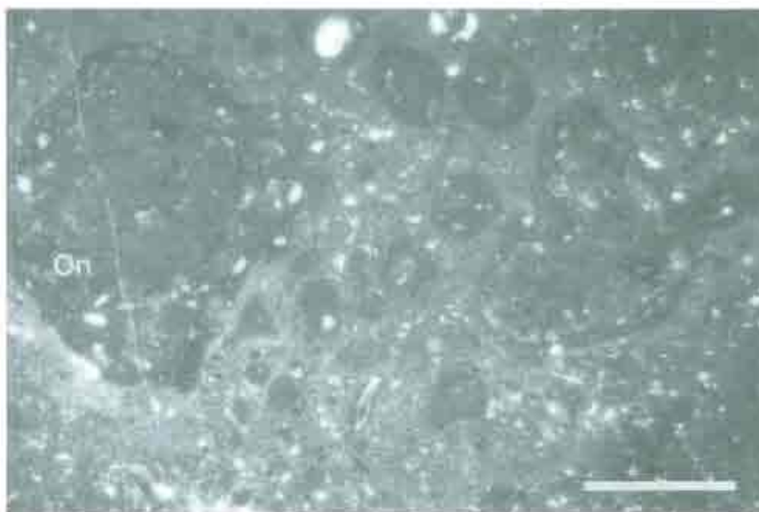
Encostramiento de granos por nubeculariidos ( Nubeculinella ) dando lugar a oncoïdes de nubeculariidos (On). Caliza grumosa oncolítica de Río Segura. (Barra 1 mm)
