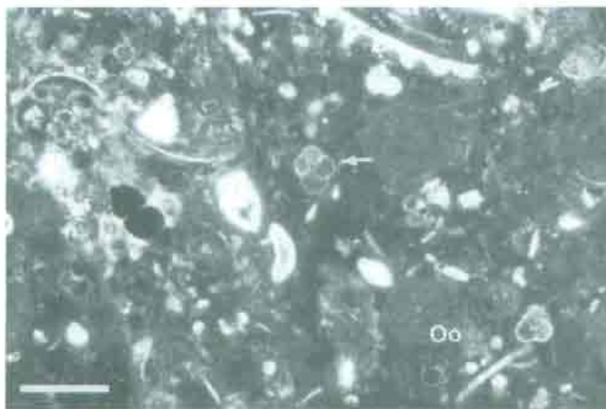
Packstone con ooides (Oo), Globuligerinas o "Protoglobigerinas" (flecha) y secciones de bivaldos. Caliza grumosa oncólítica roja de Río Segura. Barra 250 micras.
