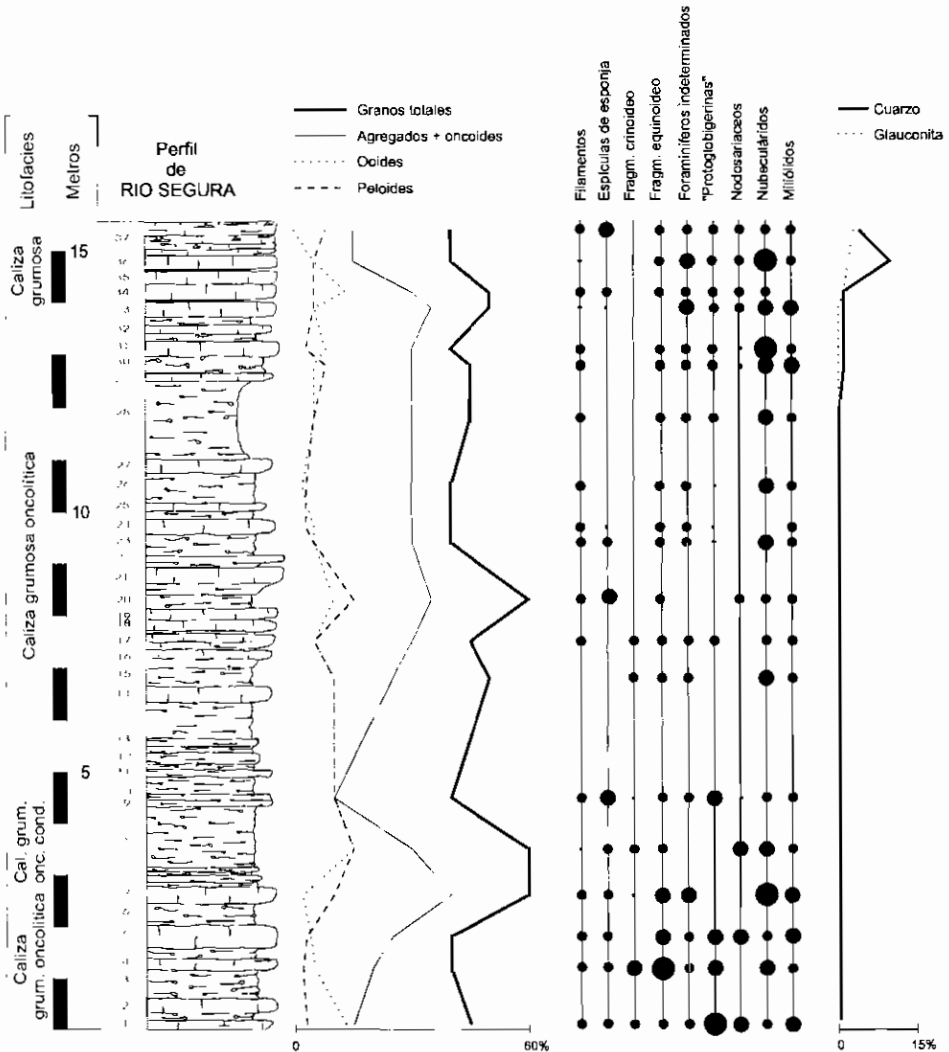
Fig. 3.- Distribución estratigráfica de los componentes reconocidos en las microfácies analizadas en el perfil de Río Segura
