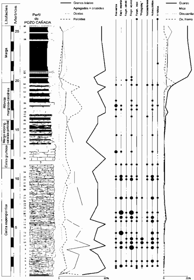
Fig. 4.- Distribución estratigráfica de los componentes reconocidos en las microfácies analizadas en el perfil de Pozo Cañada
