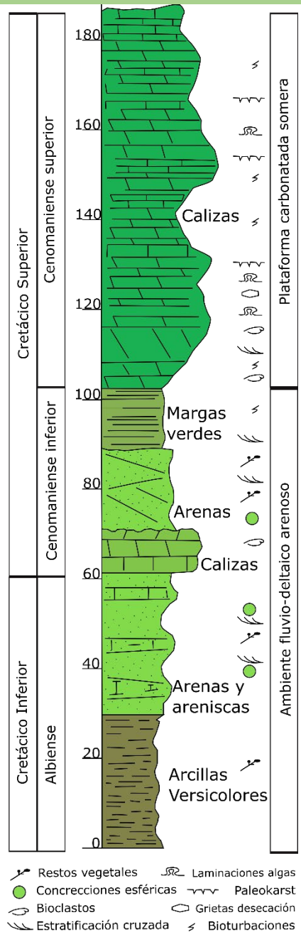
Figura 2. Serie estratigráfica del entorno de Chinchilla. Todo estos sedimentos se depositaron entre hace 113 Ma (inicio del Albiense) y 94 Ma (finales del Cenomanense).
