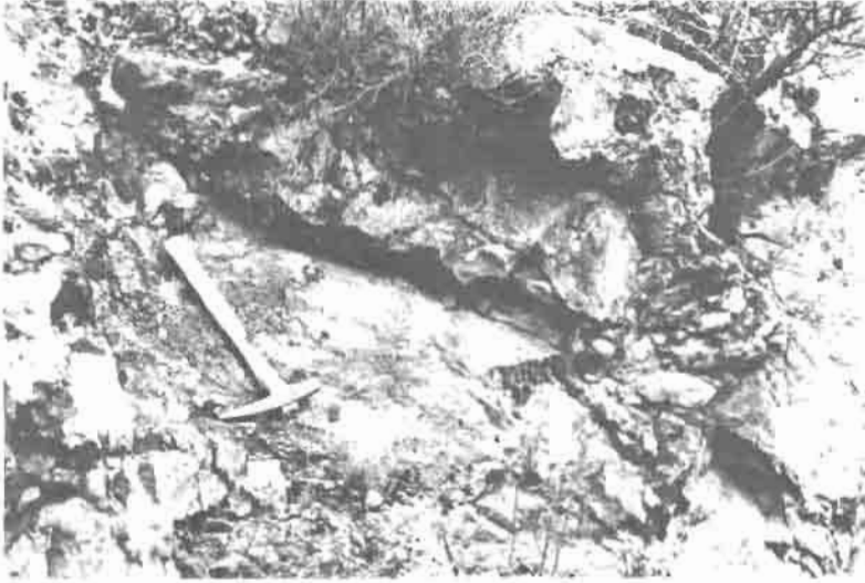
Fotog. n.º 8: Yacimiento de hematitas en la Sierra de la Higuera: Fractura donde se aloja parte de la mineralización.
