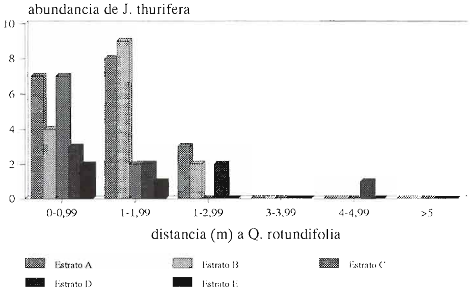
Figura 3: Número de individuos de Juniperus thurifera encontrados a diferentes distancias en relación a pies de Pinus pinea , según diferentes estratos de altura.
