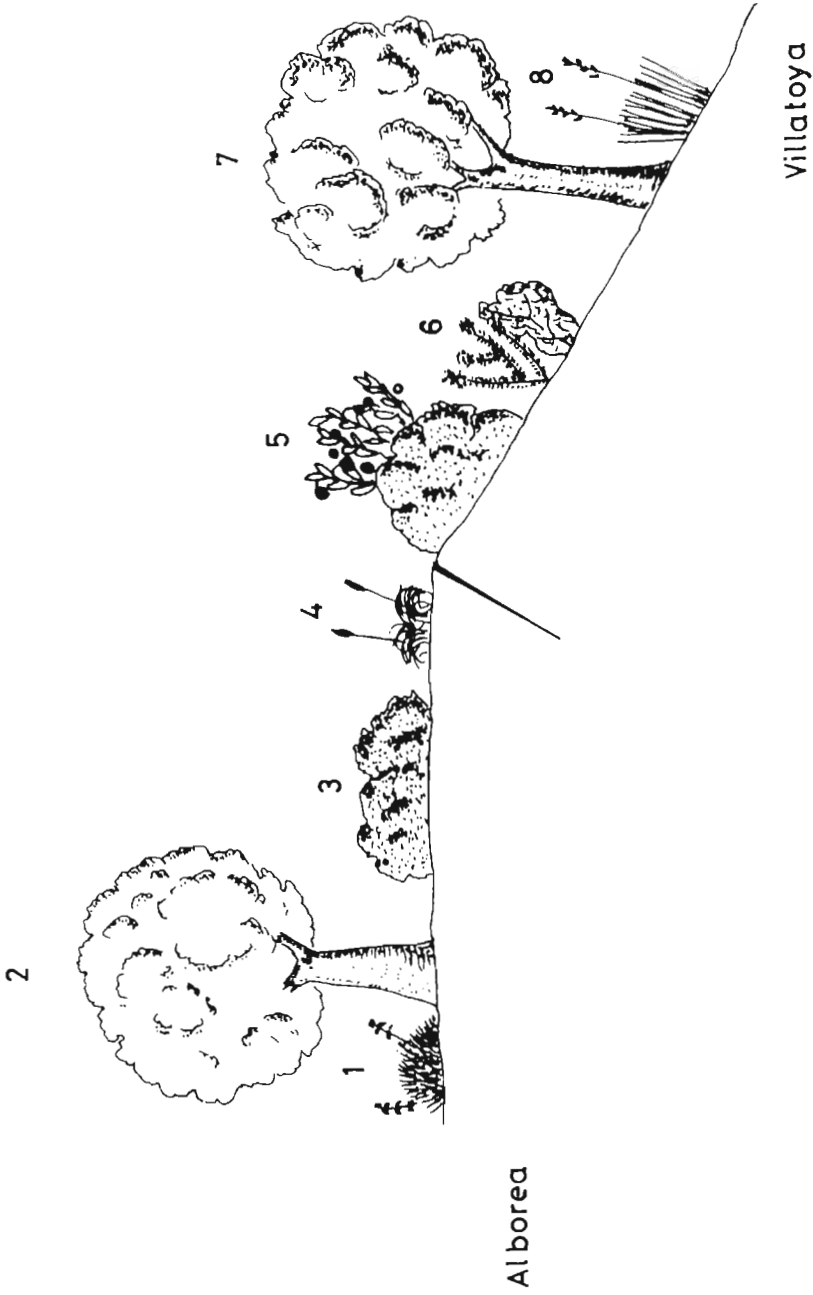
Figura 10: Corte esquemático de vegetación entre Alborea (distrito Albacetense) y Villatoya (distrito Cofrentino): 1. Matorral con marisuela y Genista mugronensis ; 2. Carrascal; 3. Coscojar; 4. Espartal; 5. Coscojar con lentiscos, madroños, durillos y bojcs; 6. Romeral con brezos; 7. Carrascal con lentiscos; 8. Pastizal de Helictotrichon filifolium .
