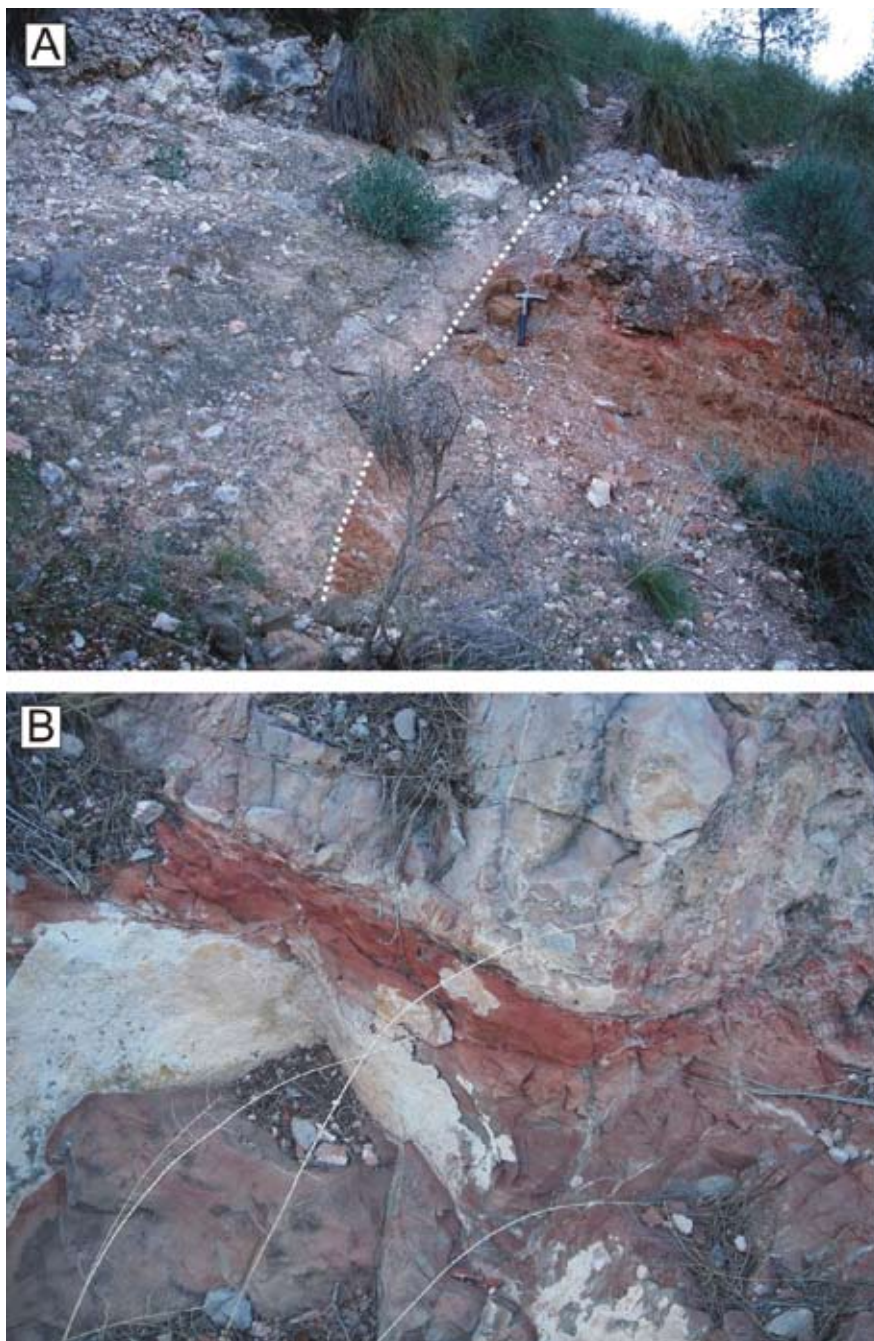
Figura 16: A. Contacto entre el complejo freatomagmático (izquierda) y la ritmita margoso-calcárea (derecha), que adquiere una tonalidad rojiza. B. Detalle de un nivel margocalizo próximo al contacto con el complejo freatomagmático.
