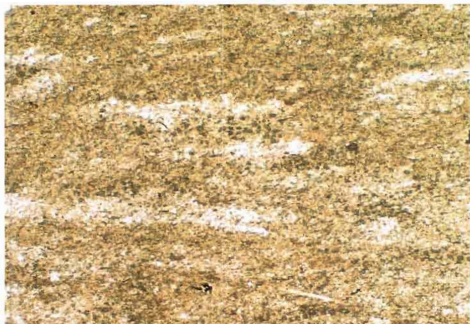
Fig. 39: Textura finamente laminada en diatomitas. Luz paralela, microscopio óptico. Cantera de Alarcón Palacios en Venta del Juez, niveles inferiores.
