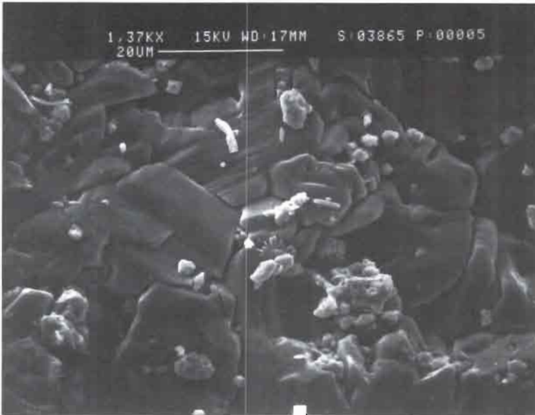
Fig. -14: Microestructura constituida por un agregado de cristales de calcita que reemplaza total o parcialmente los niveles diatomíficos. Nótese la existencia de una frústula muy disuelta en el sector central de la fotografía. Niveles infrayacentes a la porcelanita inferior aflorante en las explotaciones de Minas del Volcán en las proximidades del pantano de Camarillas. Imagen de Microscopía Electrónica de Barrido.
