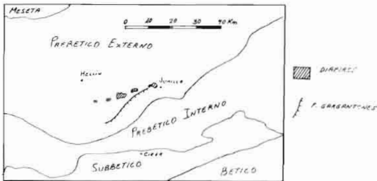
ESQUEMA — 1 — GEOLOGICO
