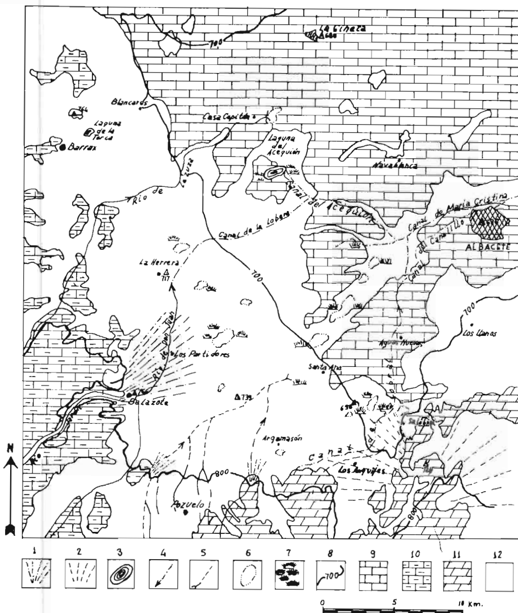
Fig. 1.— Esquema morfolitológico del sector W y SW de Albacete.
