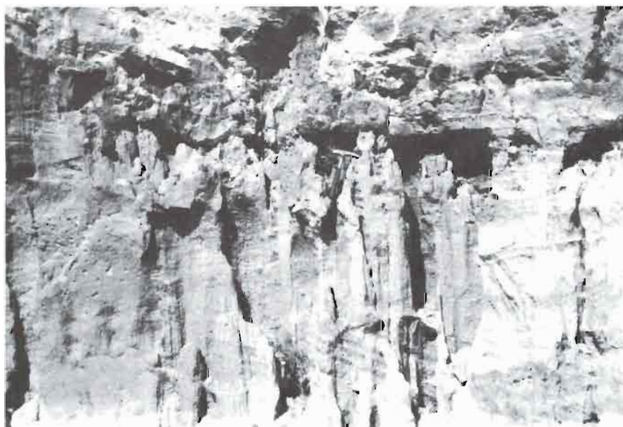
Foto 14: Erosión en chimeneas. 7.ª Parada.
