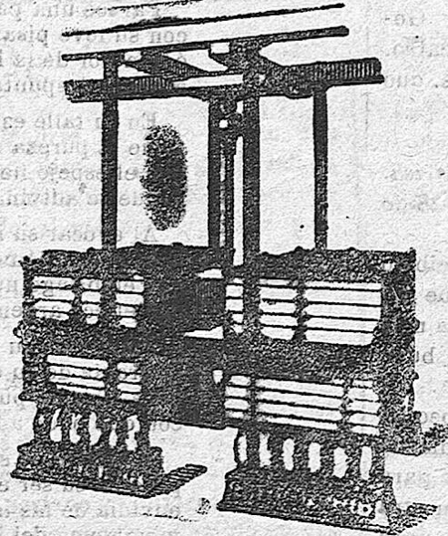
Nuevo plansichter de libre oscilación equilibrio automático. — Privilegio Buhler.
