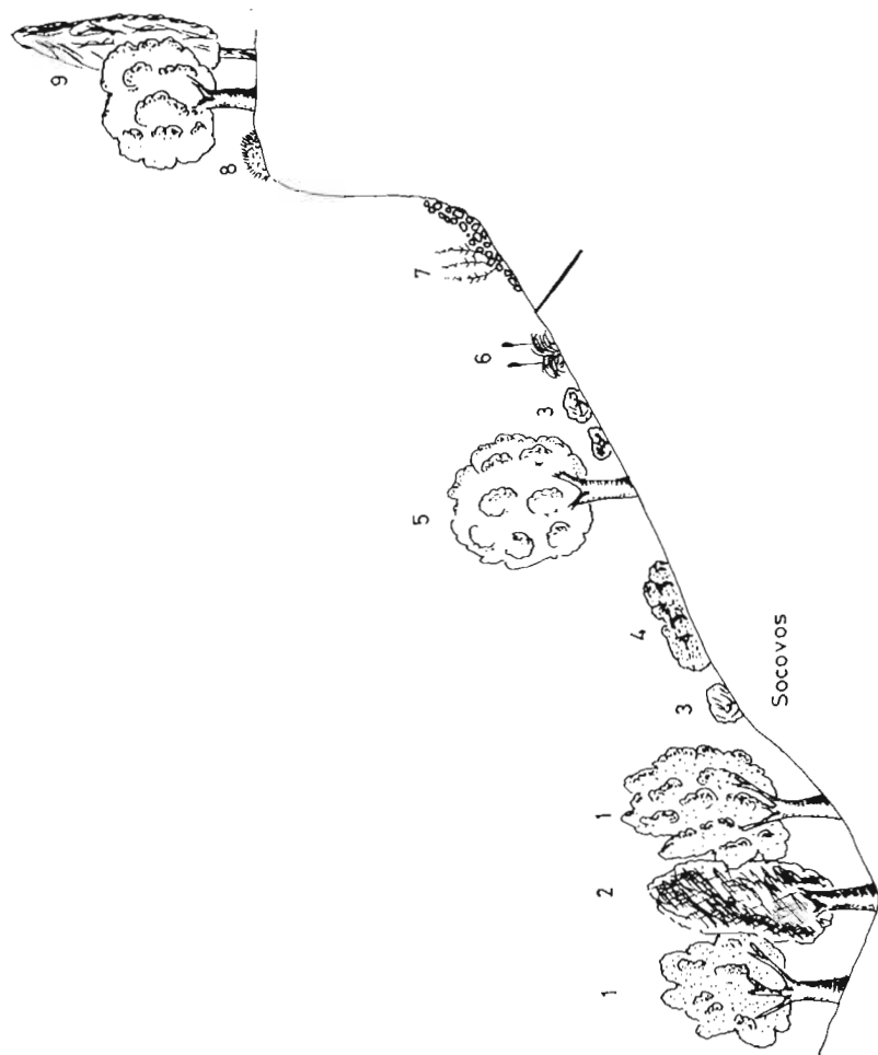
Figura 12: Corte esquemático de vegetación entre Socovos (distrito Jumillano-Socovense) y el Calar de Socovos (distrito Nerpio-Moratallense): 1. Robledal; 2. Olmedas y zarzales; 3. Romerales con Thymus funkii ; 4. Coscojar; 5. Carrascal; 6. Espartal; 7. Matorral de gleras nitrificadas con Nepeta nepetella ; 8. Carrascal con sabina albar; 9. Carrascal supramediterráneo dolomítico.
